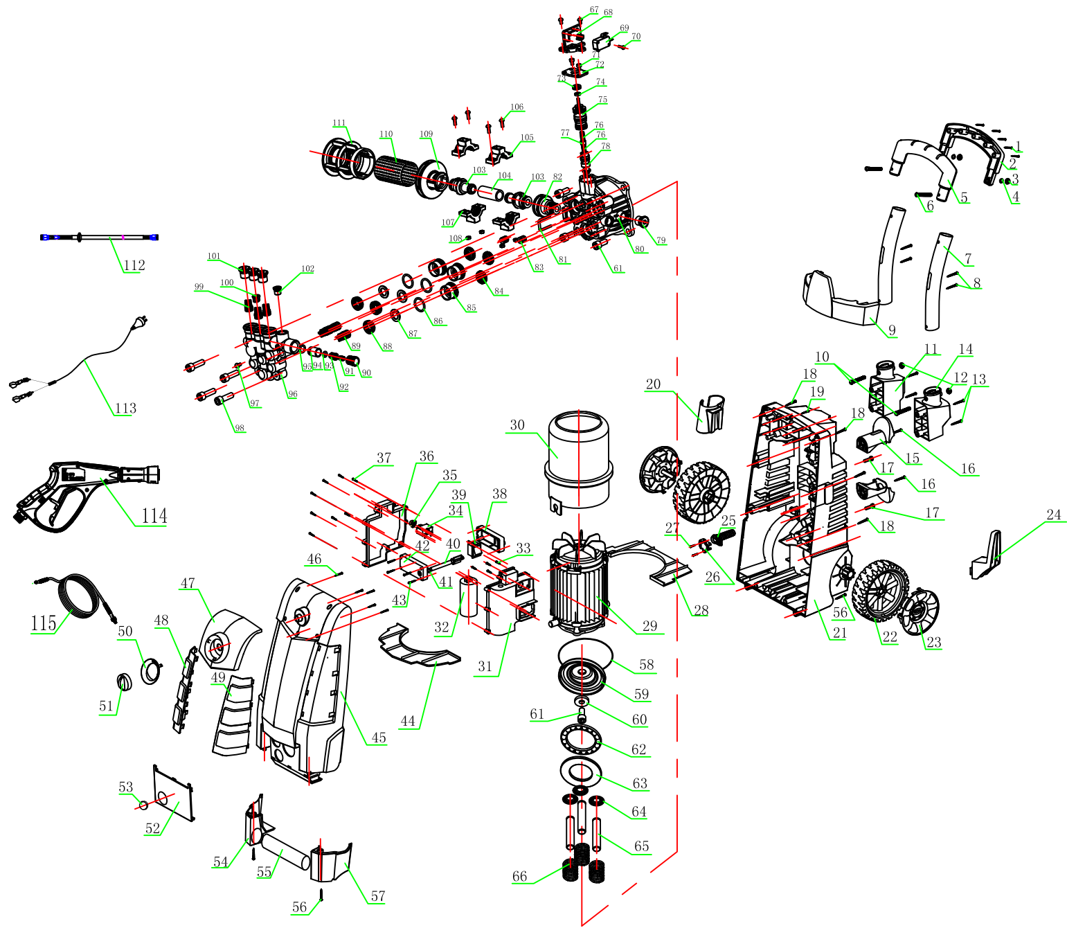
A9结构图
