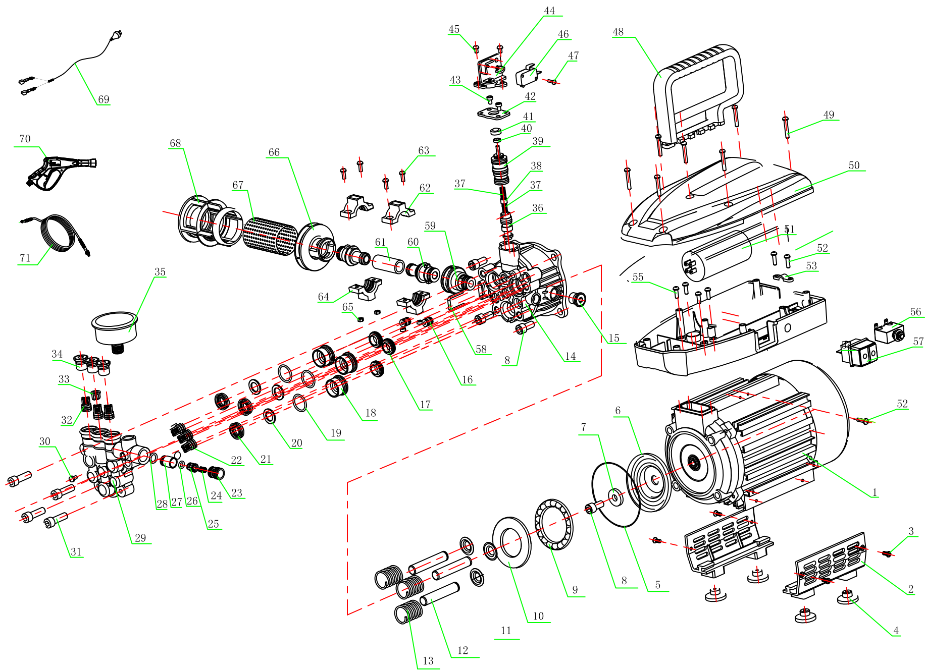
A7结构图
